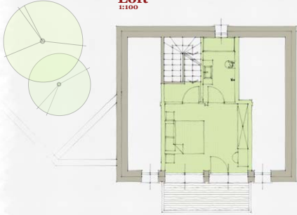
Loft 1:100
