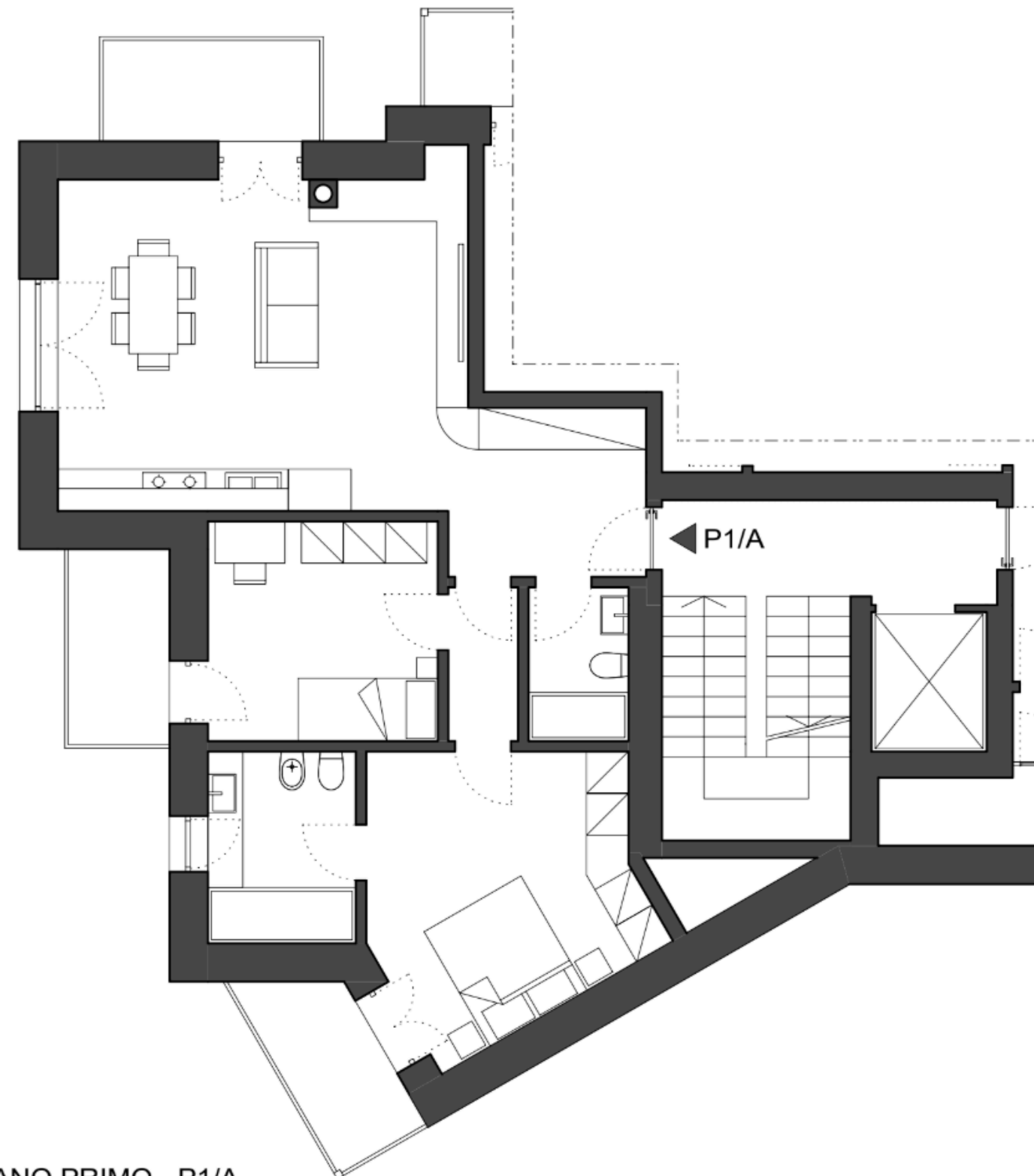
PIANO PRIMO - P1/A
